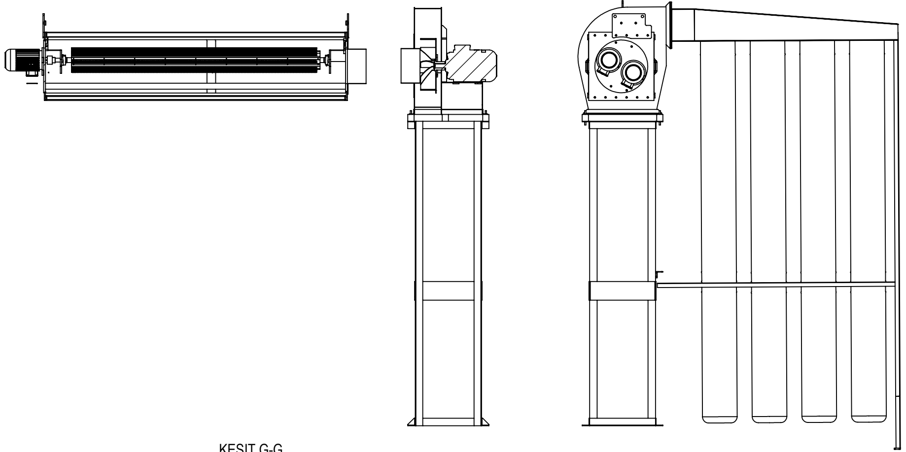
KESİT G-G ÖLÇEK 1 : 30
